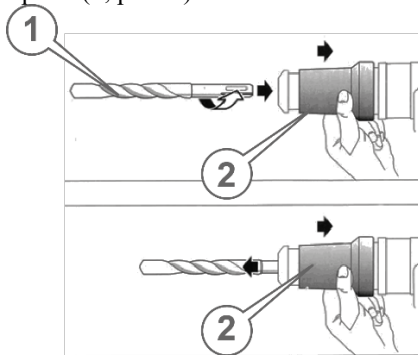
Рисунок 3. Схема встановлення/вилучення змінного кінцевого інструмента.
