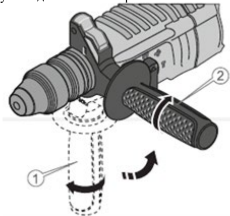
Рисунок 2. Схема налаштування допоміжного руків'я.
